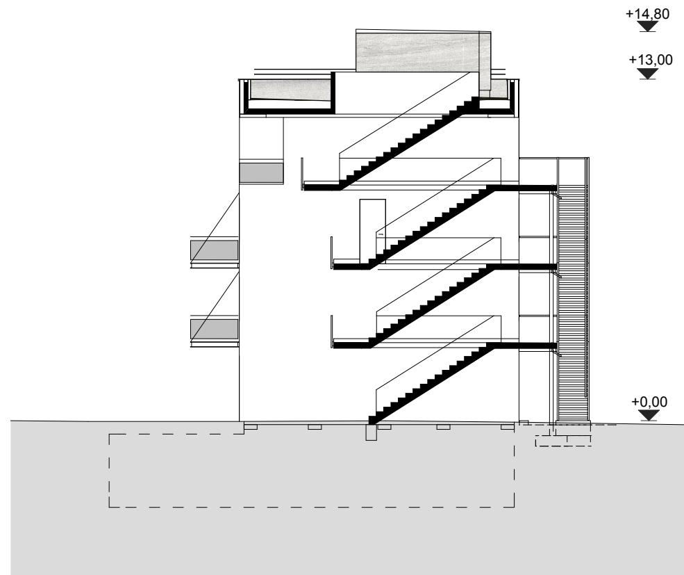
Querschnitt Treppenhaus
