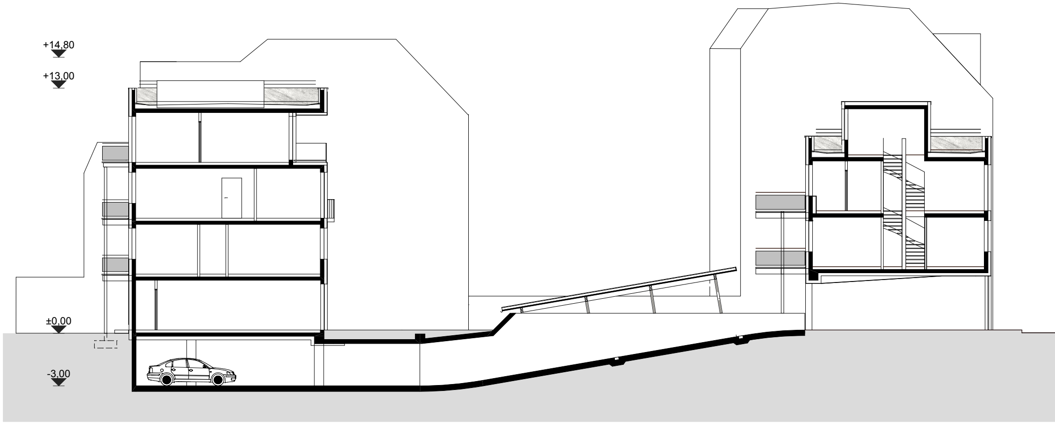
Querschnitt Tiefgarage
