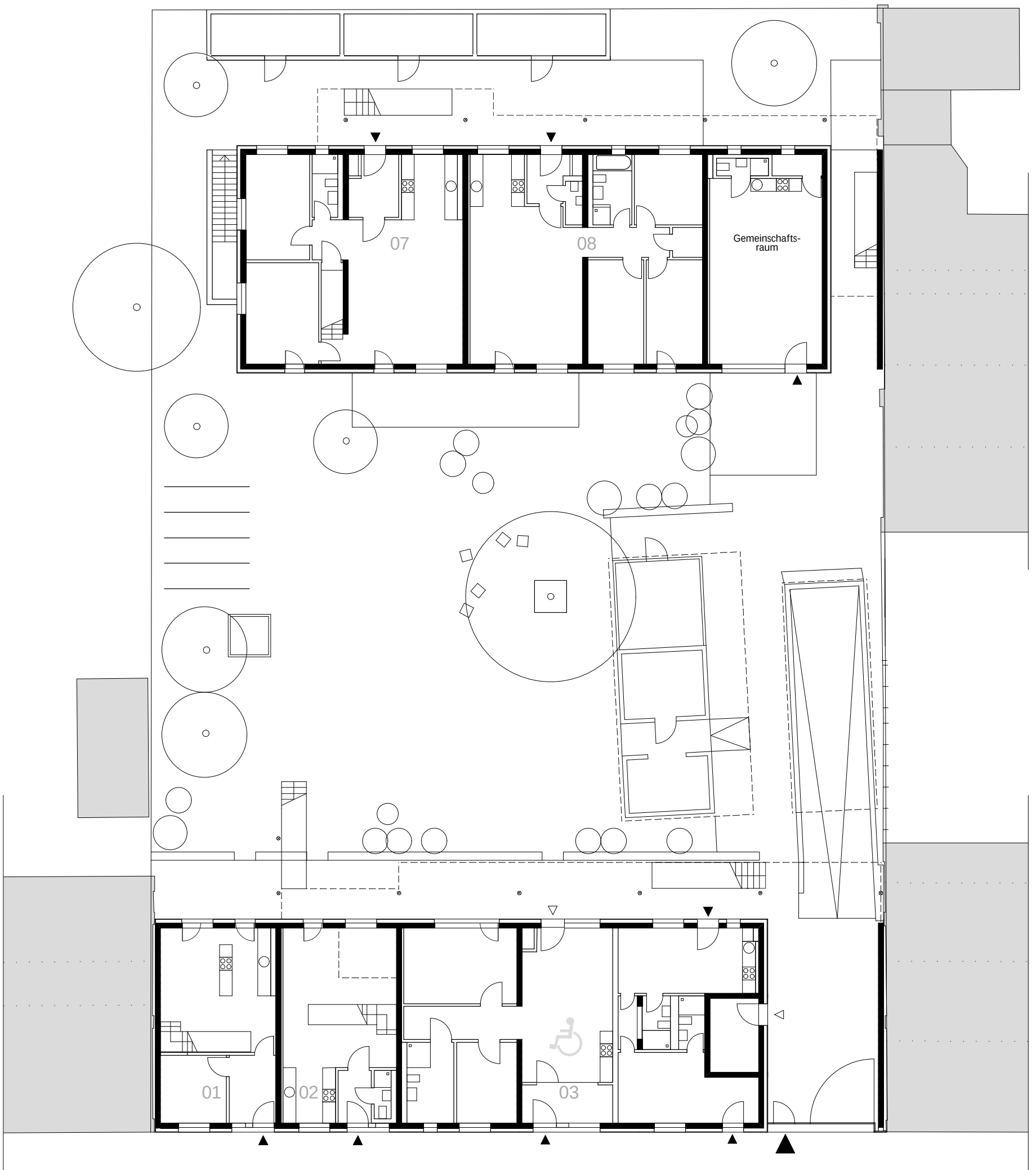
Erdgeschoss
